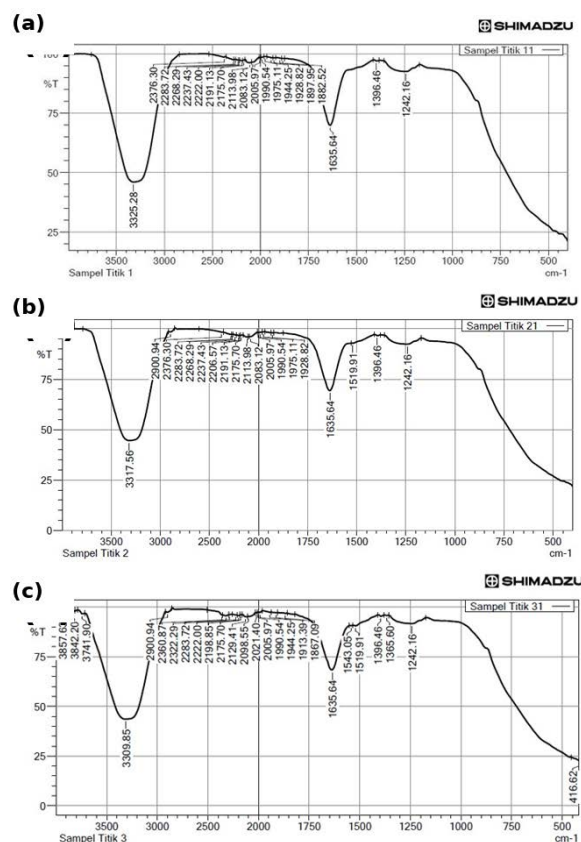
Gambar 2. Spektrum FTIR Mikroplastik pada Sampel Air Waduk Sermo: (a) Titik 1 (Inlet Sungai), (b) Titik 2 (Tengah Waduk), Dan (c) Titik 3 (Inlet PDAM)
