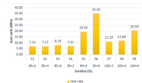
Gambar 1. Nilai rata-rata uji kuat tarik bioplastik nata de cassava terhadap konsentrasi sorbitol
